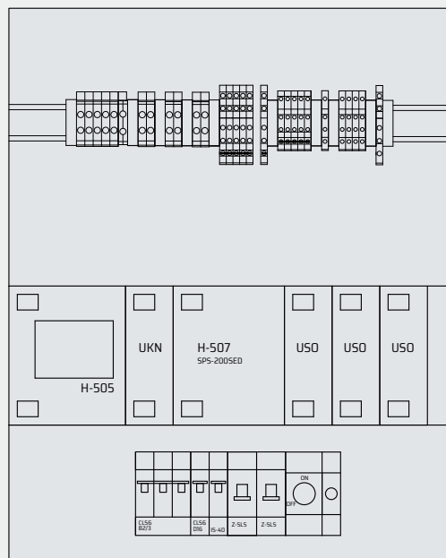
HVCBS 12U-06
