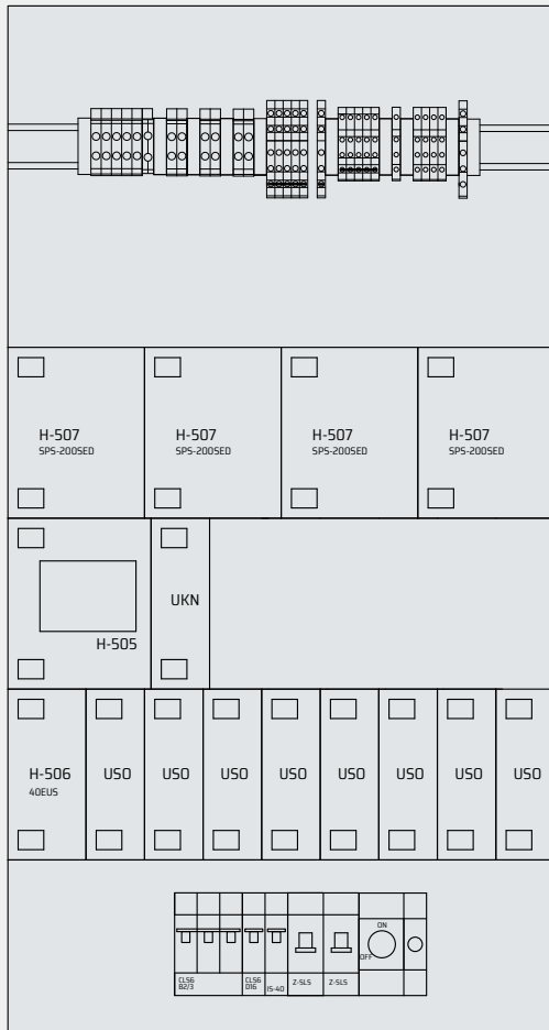
HVCBS 18U-16'''
